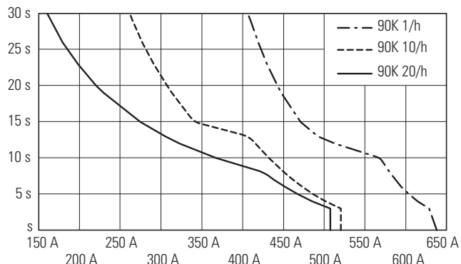
DS7-34...SX160N0-...
