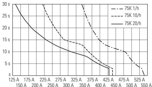
DS7-34...SX200N0-...
