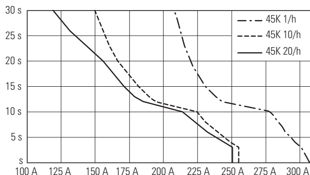
DS7-34...SX135N0-...
