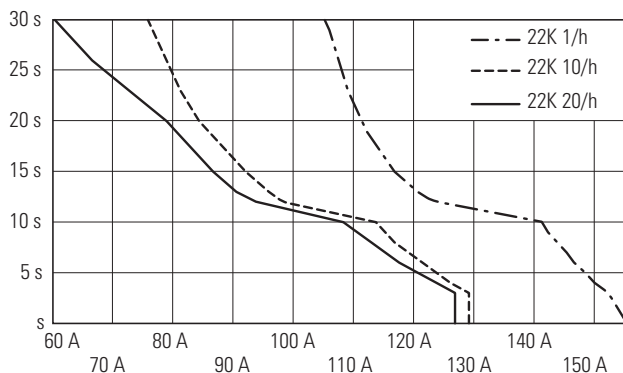
DS7-34...SX070N0-...
