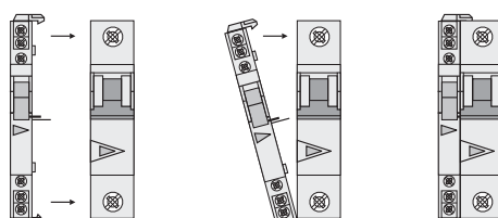
安装示例：ZP-NHK+MCB
