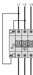
接线示例： Z-USA/400 + Z-MS
