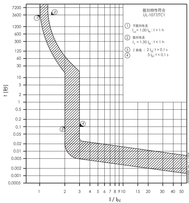
Z 曲线特性 - UL1077
