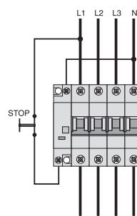
接线示例： Z-USA/230 + MCB
