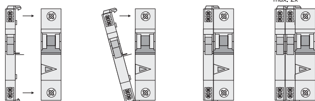
安装示例：ZP-IHK/(ZP-WHK)+MCB
