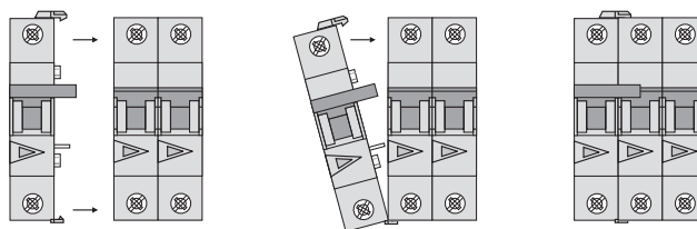
安装示例: ZP-ASA + MCB
