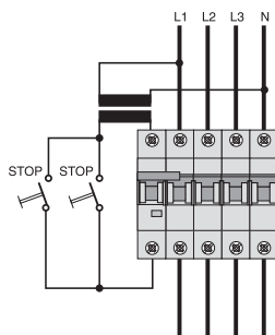
接线示例24 V
