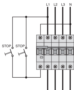
接线示例230 V
