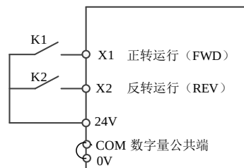
PNP型接法
