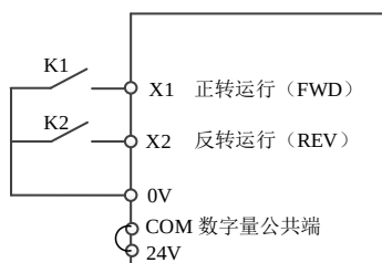
NPN型接法
