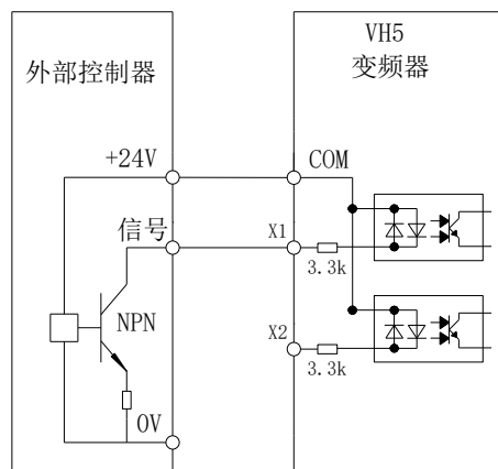
使用外部24V电源的漏型接线方法
