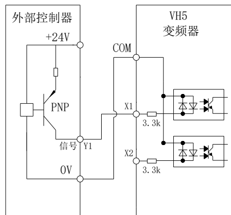
使用外部24V电源的源型接线方法
